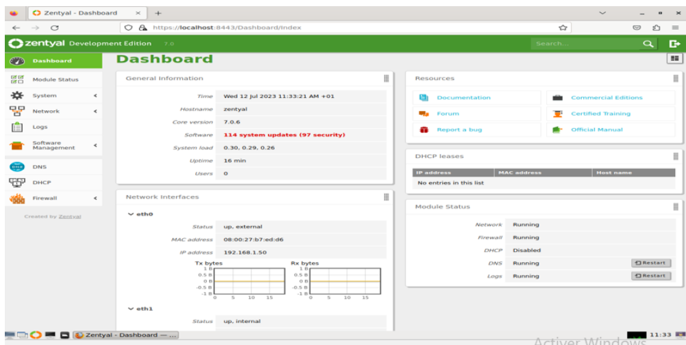
Figure 72: zentyal UI
